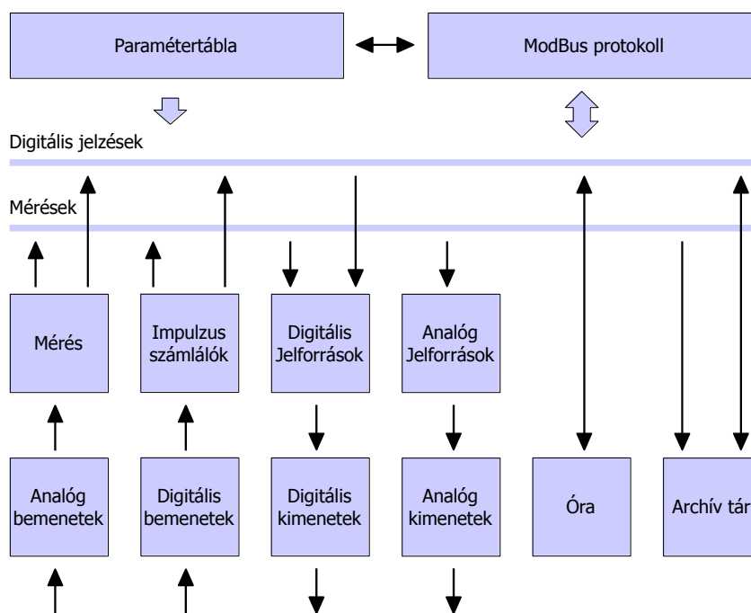
2.11. ábra Szoftver blokkvázlat
