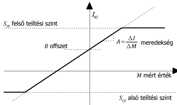
2.20. ábra. Analóg kimeneti karakterisztika
