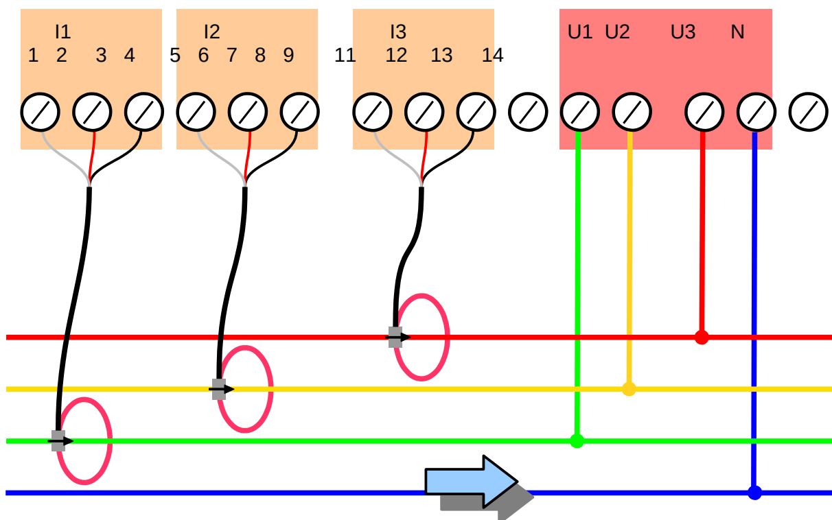
Teljesítményáramlás referenciáirány 2.10. ábra: Bekötés flexibilis áramváltókkal
