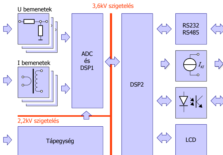
2.1. ábra: Készülék hardver elvi felépítése
