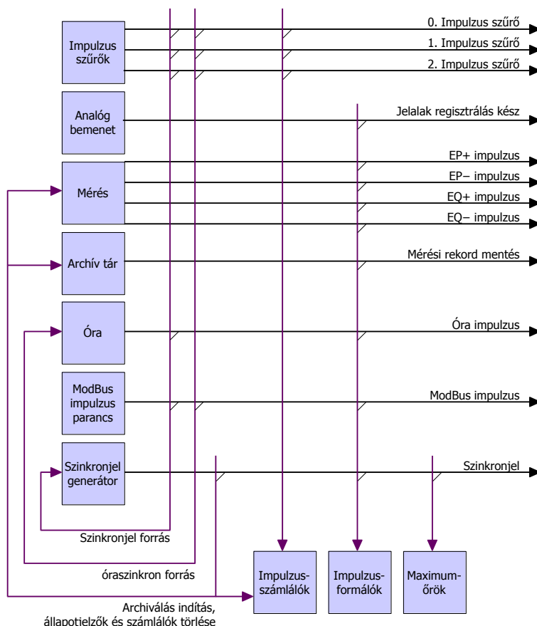
2.12. ábra. Digitális jelzések
