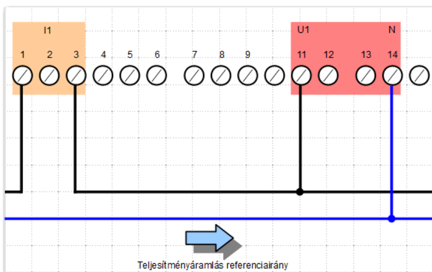
2.5. ábra: TMTG-1X direkt bekötés
