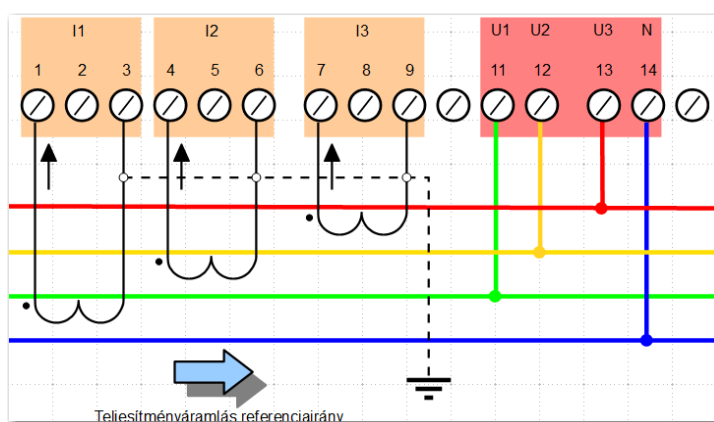
2.8. ábra: TMTG-3X áramváltós bekötés
