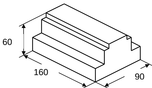
2.20. ábra: Készülék méretei
