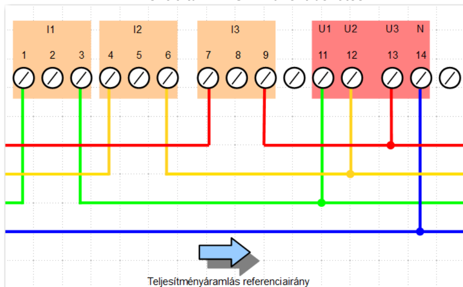
2.5. ábra: TMTG-1X direkt bekötés
