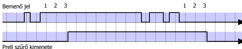
2.13. ábra: Prellszűrő működése N_{PR}=3 esetén
