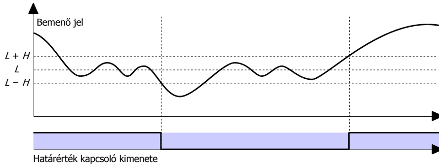
2.16. ábra: Határérték kapcsolók működése
