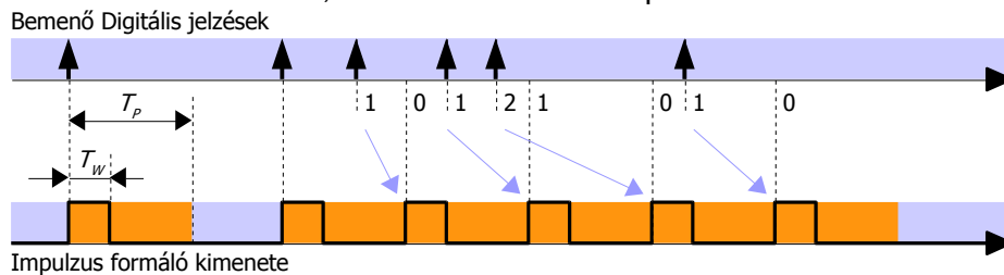
2.17. ábra. Impulzusformálók működése
