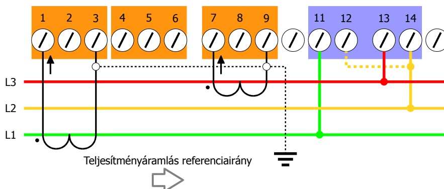
2.9. ábra: Bekötés Aron kapcsolású mérés esetén
