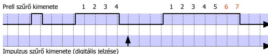
2.14. ábra: Impulzus szűrő T_{IMIN}=2ms és T_{IMAX}=5ms esetén
