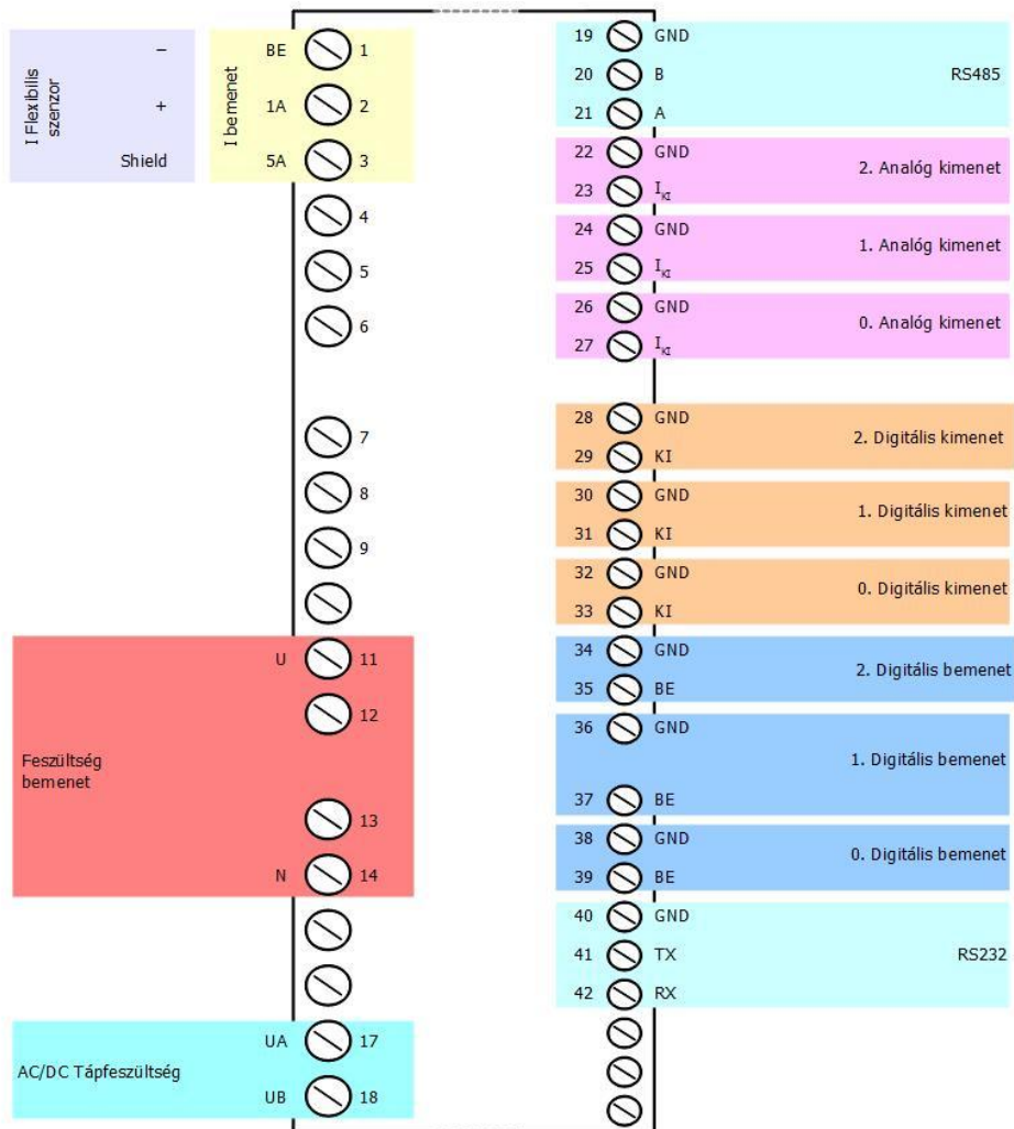
2.3. ábra: TMTG-1X Sorkapocs kiosztás
