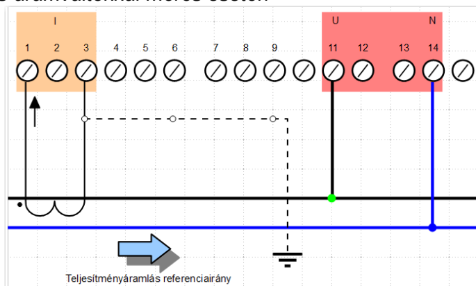
2.7. ábra: TMTG-1X áramváltós bekötés
