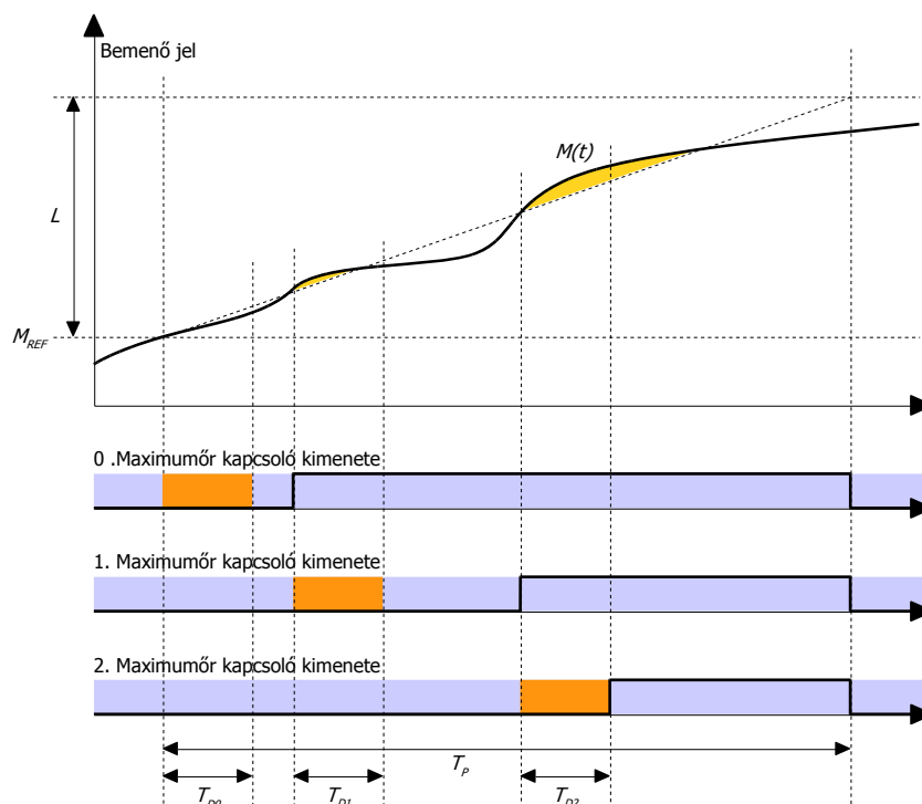
2.19. ábra. Maximumörök működése kaszkád üzemmódban
