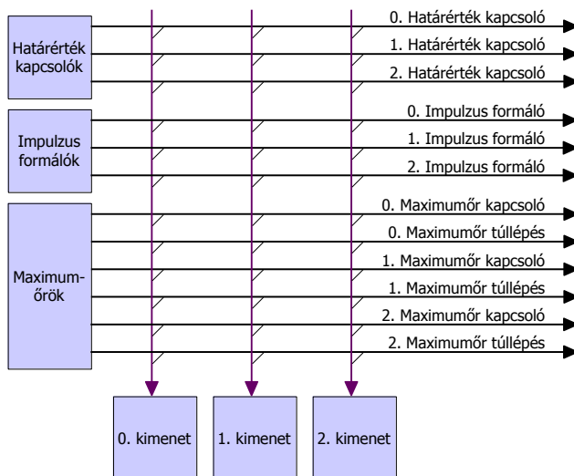
2.15. ábra: Digitális jelforrások és kimenetek
