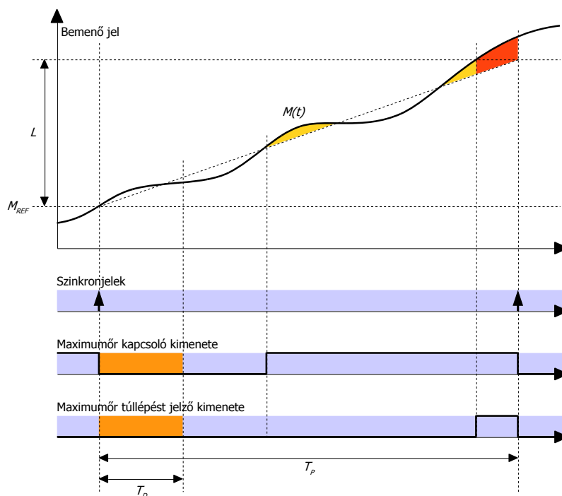
2.19. ábra. Maximumörök működése önálló üzemmódban
